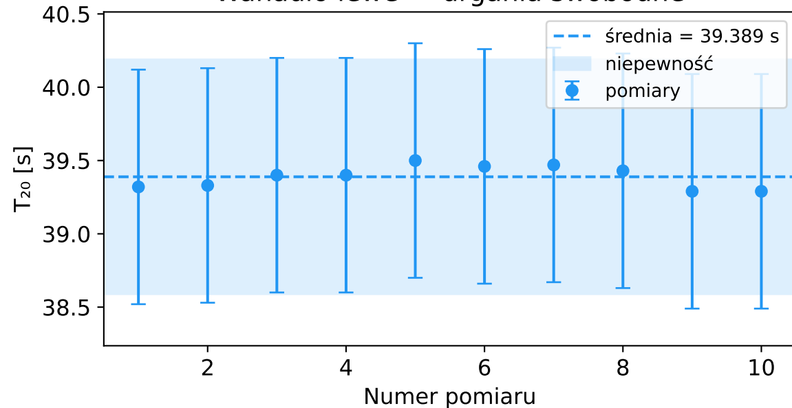
Wahadło lewe — drgania swobodne
